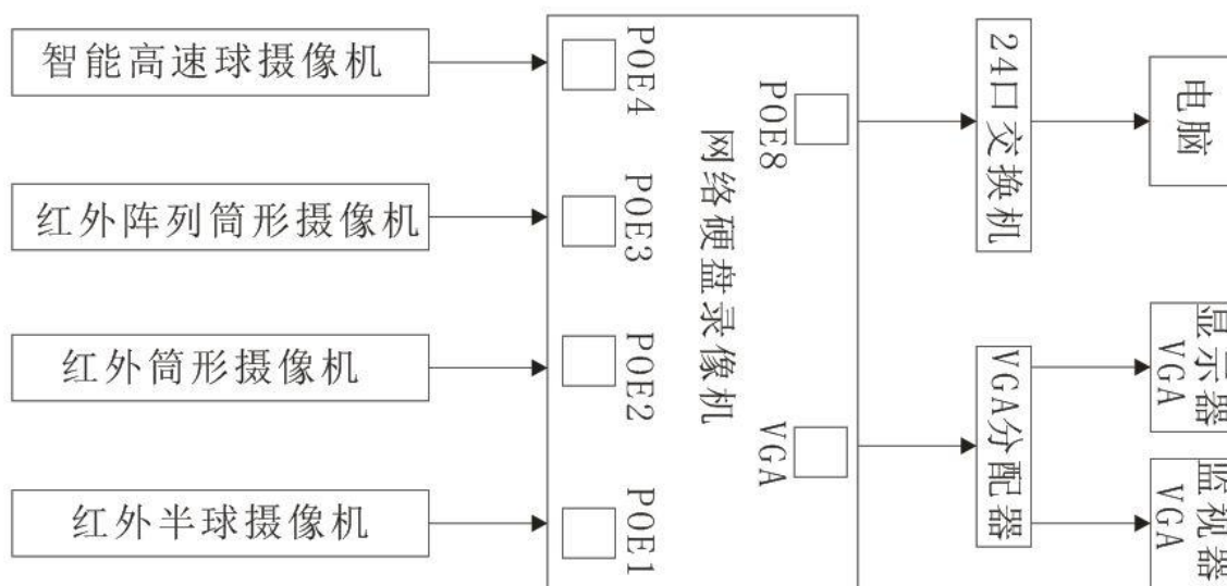
图3网络摄像机外接线示意图
