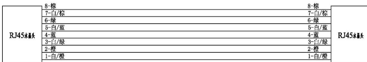
图2 网络视频监控子系统的网线
