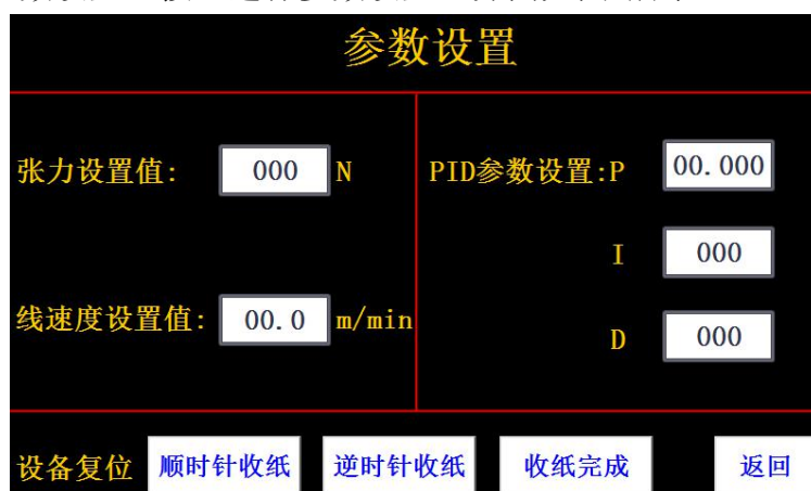
图7 张力系统参数设置界面
