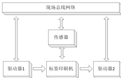
图2 标签印刷生产线的控制流程
