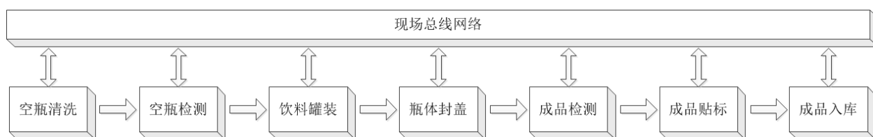
图1 饮料罐装生产线的工艺流程
