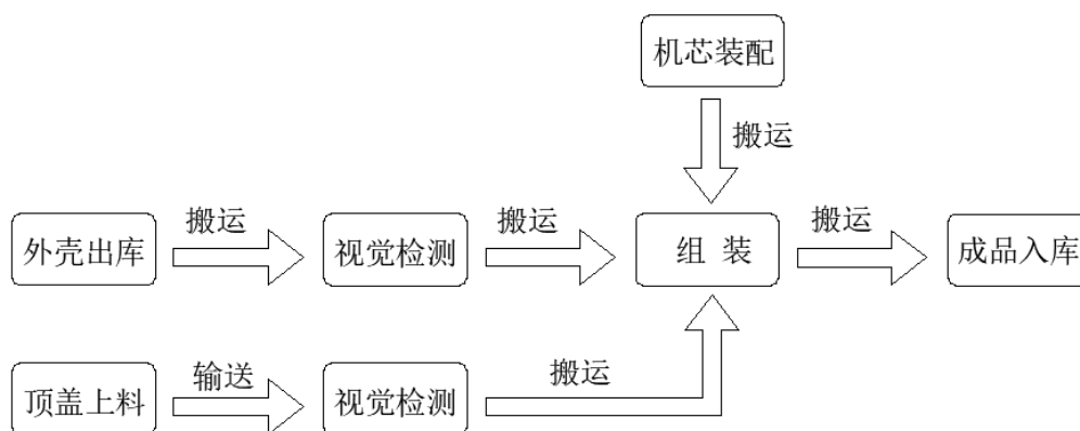
图 1 工件装配生产工艺流程
