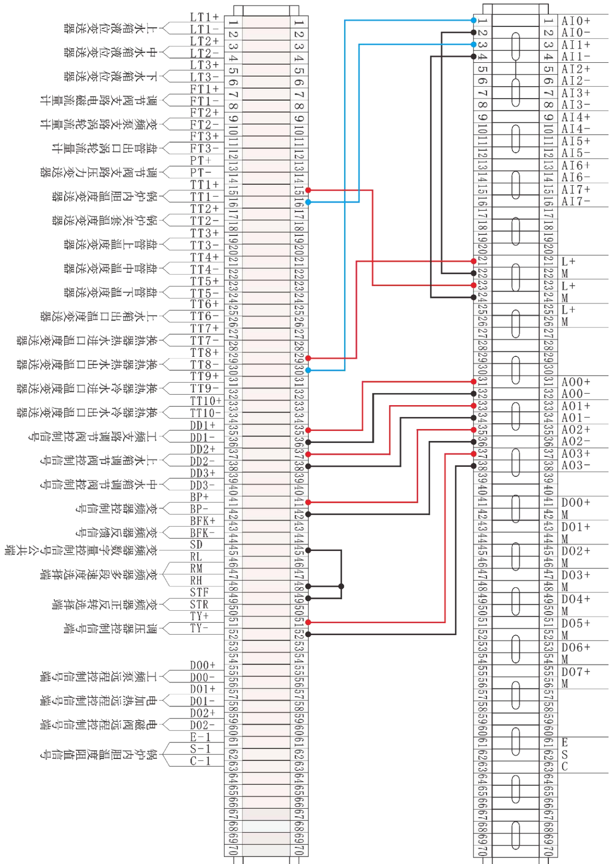
a、PLC 控制系统接线图
