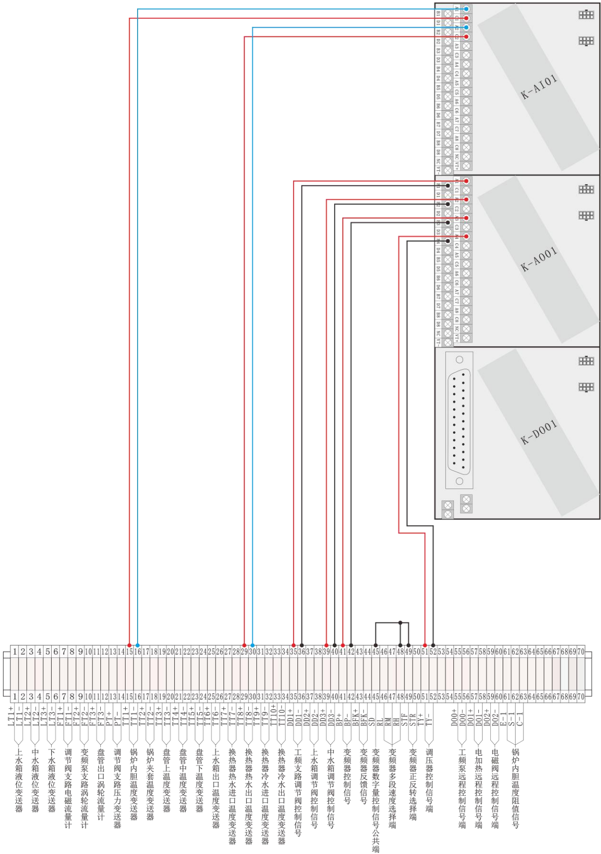
b、DCS 控制系统接线图 图 2 控制系统接线图
