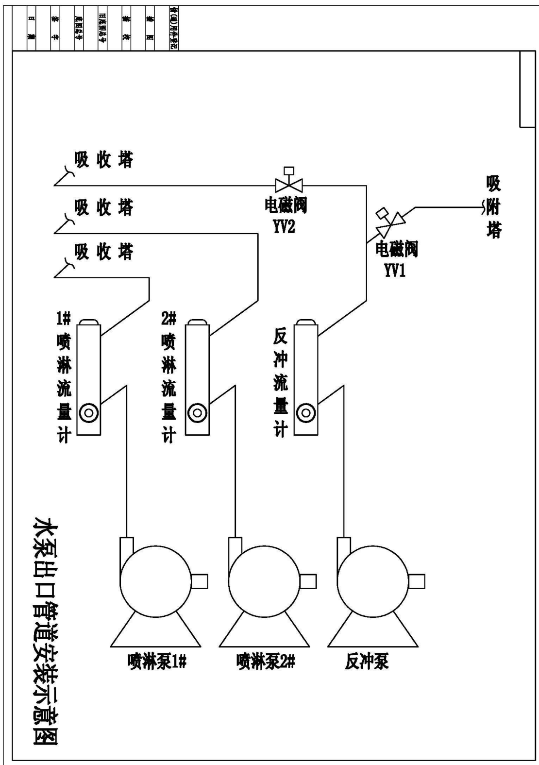
附图 2：水泵出口管道安装图
