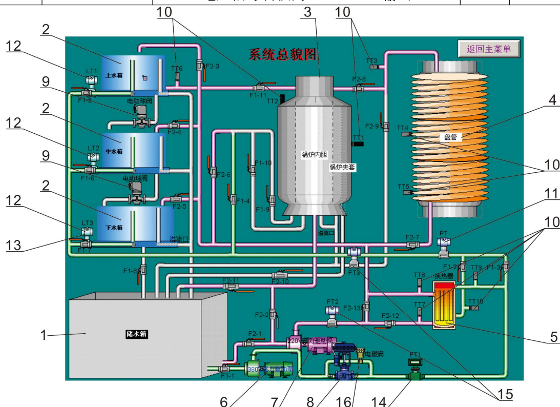
1-储水箱、2-有机玻璃液位水箱、3-带夹套不锈钢锅炉、4-盘管、5-板式换热器、6-工频磁力驱动泵、7-变频磁力驱动泵、8-智能直行程电动调节阀、9-电动调节球阀、10-温度传感器、11-管道压力变送器、12-扩散硅液位变送器、13-PA 总线液位变送器、14-电磁流量计、15-涡轮流量计、16-电磁阀
