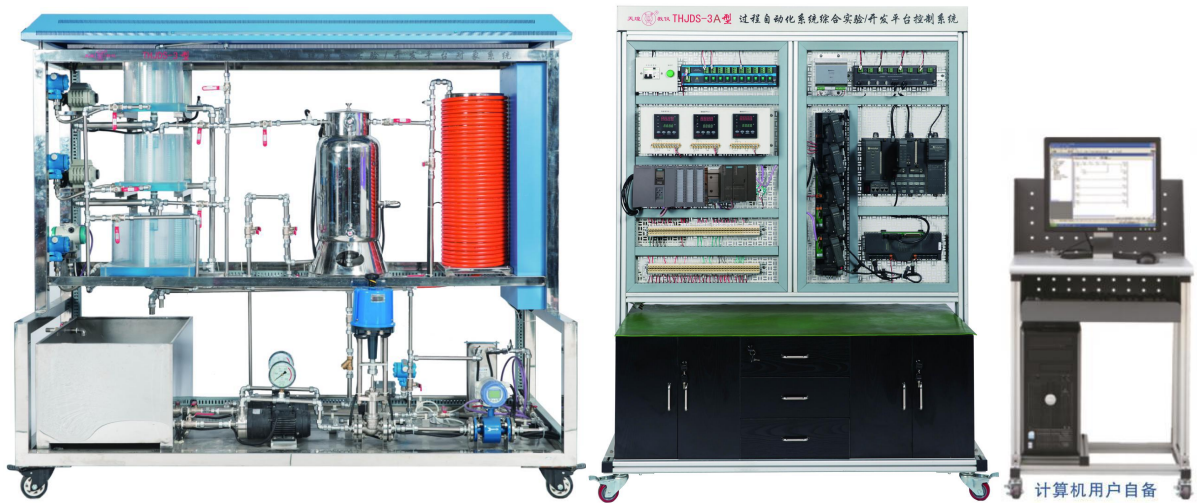
图 1 赛项平台（过程自动化系统综合实验/开发平台）
