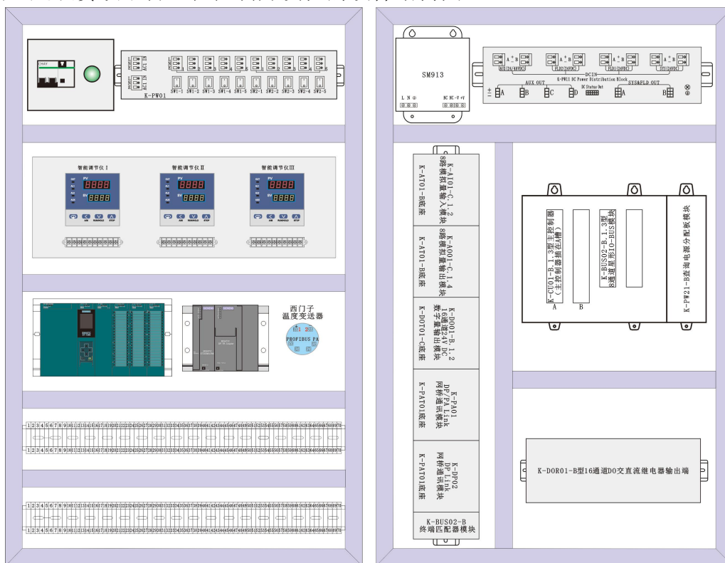
图 2 赛项平台控制屏硬件结构图
